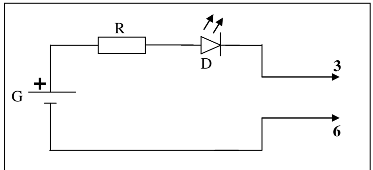
الرسم 1: رسم مقنّن (مبسّط) للدارة الكهربائية لرانز إستمرارية التيار الكهربائي
